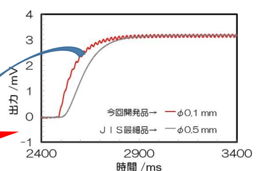
図3. 応答性試験の結果
