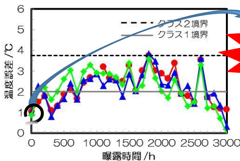
図2. 500^\circ\text{C} 曝露試験の結果
